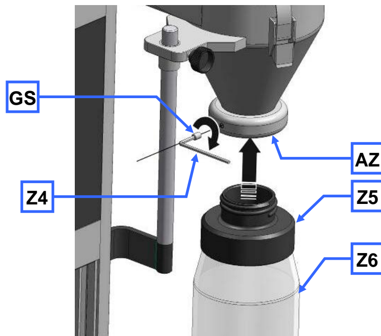
Fig. 10: inserimento dell'adattatore per le bottiglie a collo largo
