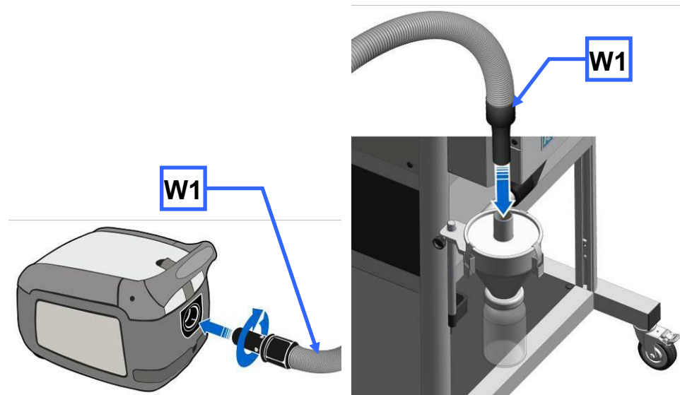
Fig. 9: collegamento dell'aspirapolvere industriale
