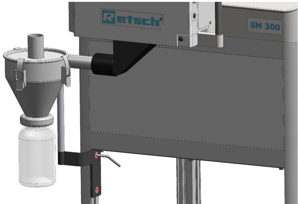
Fig. 8: ciclone assemblato
