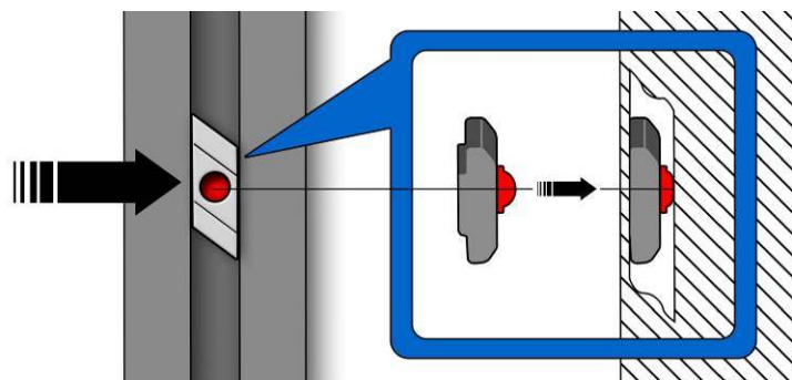
Fig. 4: inserimento della chiocciola
