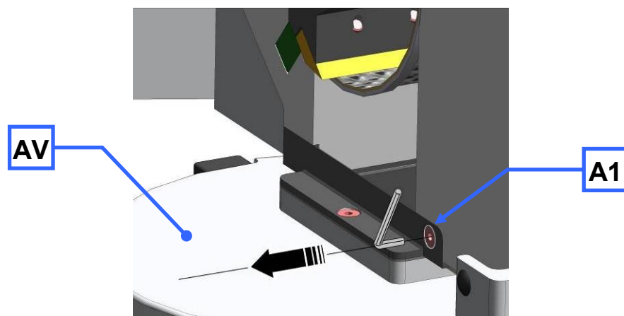
Figure 1 : Suppression de la bride d'évacuation
