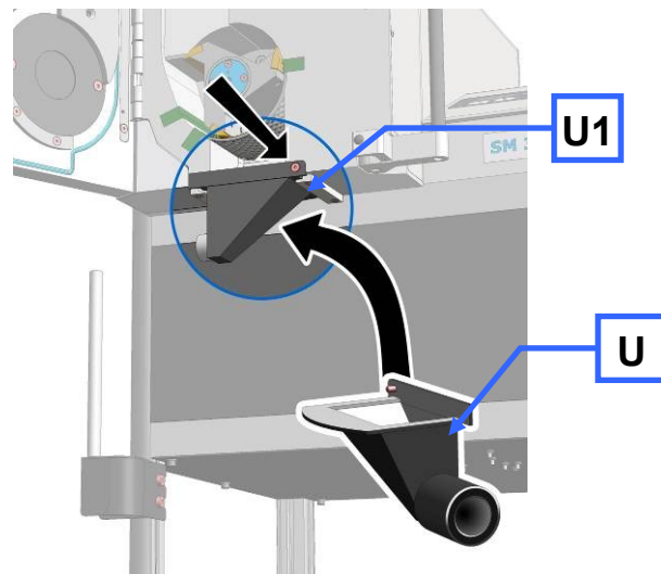
Figure 2 : Fixation de la bride d'évacuation
