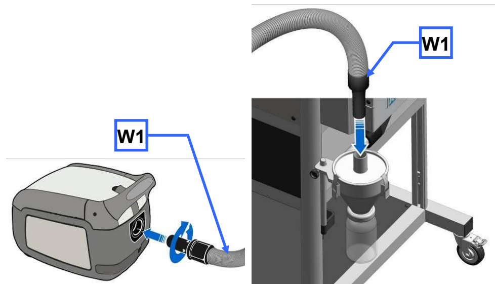
Figure 9 : Raccordement de l'aspirateur industriel
