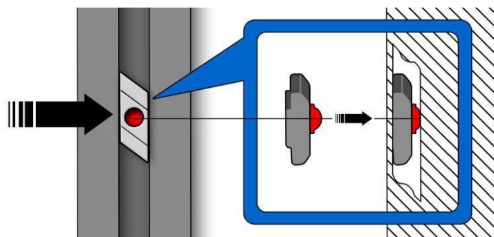
Figure 4 : Mise en place de la clavette rainurée
