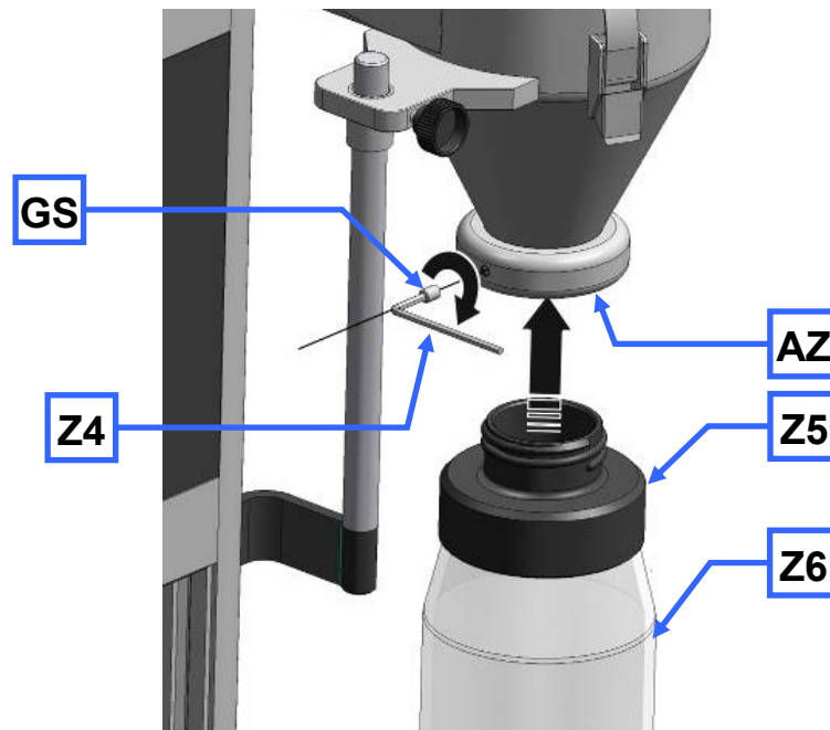
Figure 10 : Mise en place de l'adaptateur pour les bouteilles à col large
